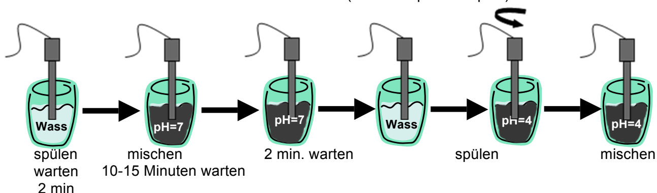
Figure 11. Kalibrierung des pH-Sensors
