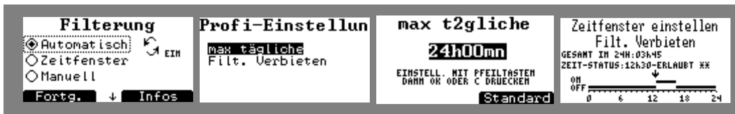
Figure 5. Programmierbildschirm der Filterung in gesteuerten Modus.
