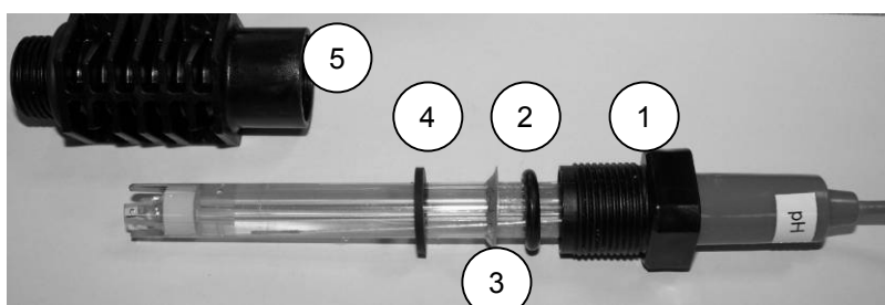
Figure 14. Platzieren der Sensorträger
