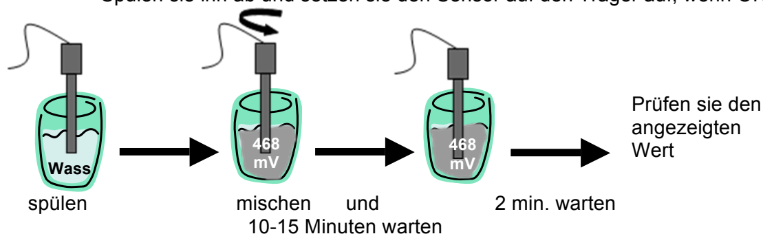
Figure 12. Verifizierung des Redox-Sensors
