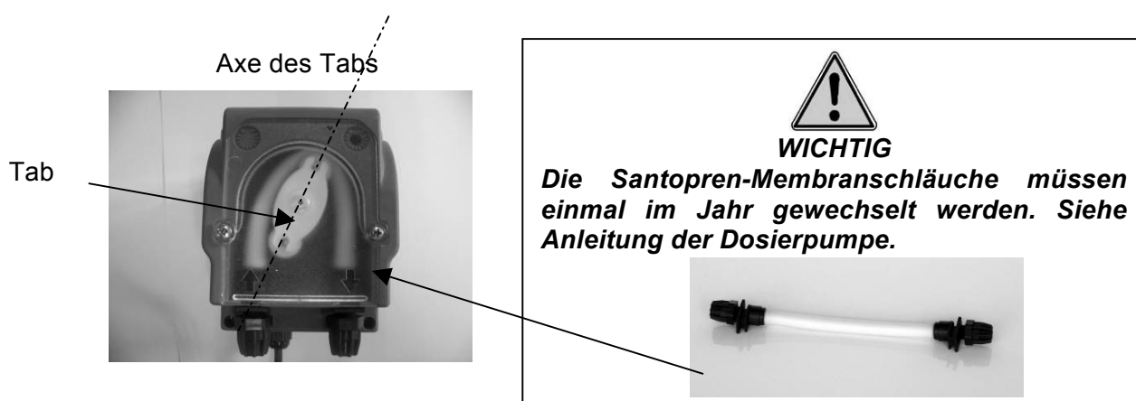
Figure 13. Dosierpumpe
