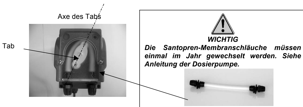
Figure 12. Dosierpumpe
